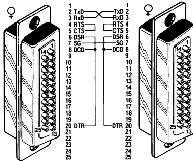
Interconnexion trifilaire DTE-DTE
