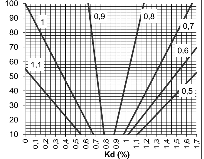
Moteur 6 et 8 pôles h ≥ 160mm
