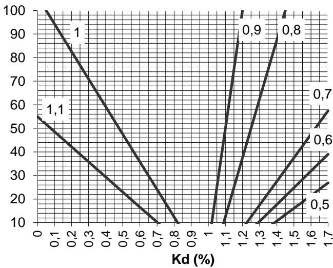
Moteur 6 et 8 pôles h ≤ 132mm
