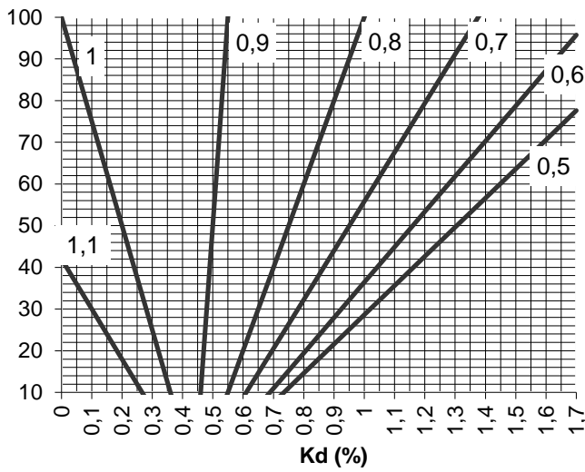
Moteur 4 pôles 1500 tr/min h ≤ 132mm
